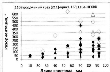
Рис. 4. Значения разориентации [°] по длине (110)-ориентированного продольного среза (211)-кристалла GeSi-168 (Рис. 5), высокоэнергетическая РД-спектроскопия (большие точки: мозаичность из полного уширения КК, малые точки: локальные разориентации внутри блоков, пустые точки: разориентации блоков, оцененные по угловым расстояниям между пиками КК).
