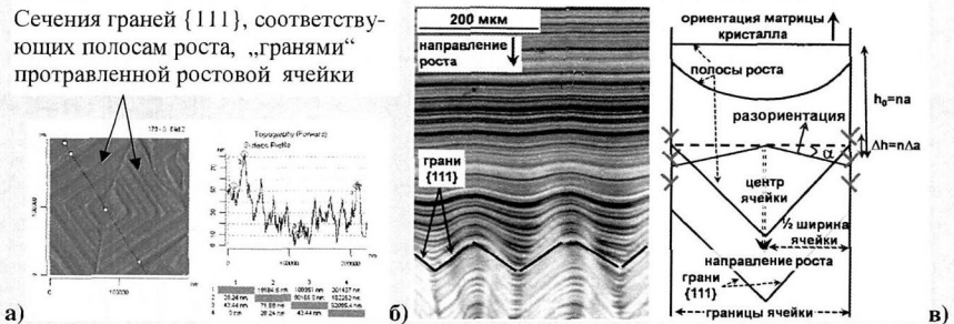
Рис. 8. а) Топография и профилометрия протравленной ростовой ячейки (100)-кристалла Ge_{1-x}Si_x (поперечный срез); наклон „граней“ ячейки \approx 100'' , б) начало образования ячеистой структуры (продольный срез); в) модель компенсации несоответствия решетки разориентацией \alpha , напряжения компенсируются дислокациями ( \perp ) в границах ячеек.
