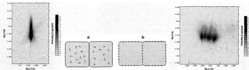
Рис. 6. КОП, поперечные сечения (211)-кристалла, отражение (422). Слева: начало кристалла, область без выраженной мозаичности. Справа: конец кристалла с ростовыми ячейками. В центре: модель распределения дислокаций при компенсации напряжений а) дислокациями в объеме ячеек либо монокристалла (сравните КОП слева), б) генерацией дислокаций в границах блоков/ростовых ячеек (сравните КОП справа).
