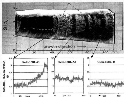
Рис. 5. Корреляция распределения Si (FTIR сверху и МРА внизу) и ячеистой структуры (селективное травление, OM) по длине продольного среза (211)-кристалла. Слева – начало, справа – конец кристалла.
