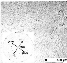
Селективное травление, ОМ: Рис. 1. Ростовые ячейки на поперечном срезе (100)-кристалла Ge_{1-x}Si_x .
