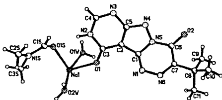
Рис. 1. Молекулярное строение соединения 49
