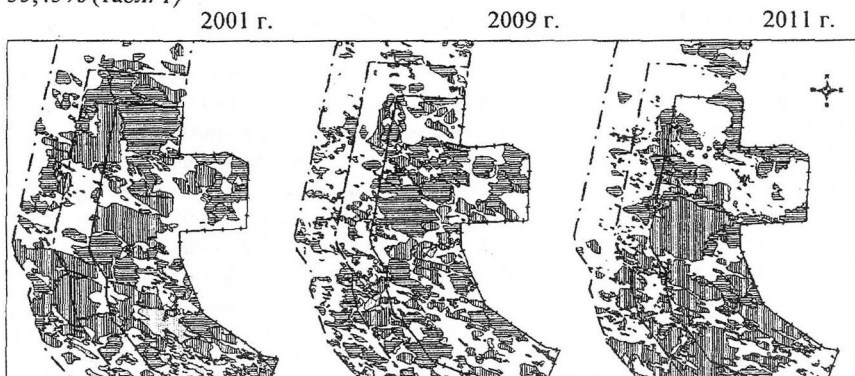
Рис. 5. Карта-схема расположения природных контуров в зонах заповедной, охранной и выпаса Яшкульского и Черноземельского районов. М 1:2,5 км (Landsat-7, ЕТМ+, 2001 г., 2009 г., 2011 г.)
