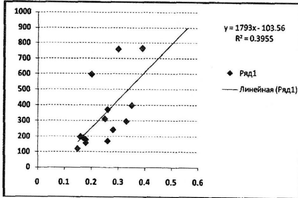
Рис. 4. Значения показателей NDVI и продуктивность сырой массы на ключевых участках заповедной, охранной и выпасаемой зон (по снимку с ИСЗ «Landsat-7», сканер ETM+, 01.06.2011)
