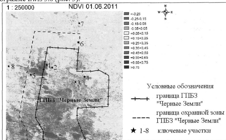
Рис. 3. Фрагмент обработанного в Ilwis 3.6 космоизображения с ИСЗ «Landsat-7» (сканер ETM+, 01.06.2011) для расчета индекса вегетации
