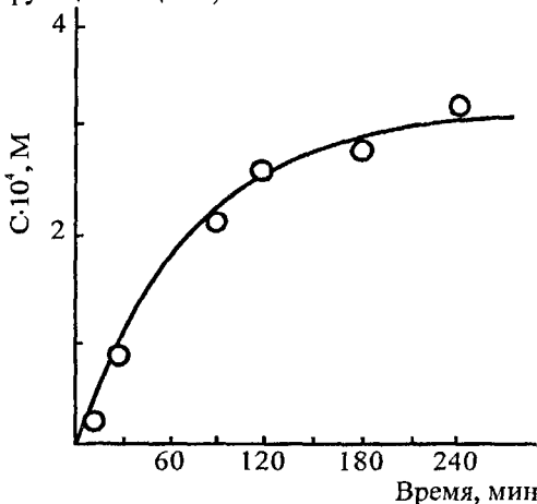
Рис. 2. Кинетическая кривая накопления пероксibuтановой кислоты в опыте взаимодействия 10.87 М бутановой кислоты с 0.01 М раствором пероксида водорода при 20^\circ\text{C} .
