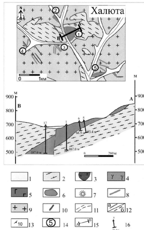
Рис. 7. Схемы геологического строения Халютинского месторождения, Аршанского и Южного проявлений карбонатитов по (Мауришин и др., 1976; Карбаинов и др., 1979; Рипп и др., 2000). 1 –алевриты, песчаники, аргиллиты (K); 2 –биогитовые, амфибол-биогитовые разнотельные граниты, граносиениты, кварцевые диориты, гнейсограниты (PZ 1 ); 3 – перидотиты (PZ 2 ); 4 – анортозиты; 5 – амфибол-пироксеновое габбро (PZ 3 ); 6 – 8 – карбонатиты: 6 – участки площадного распространения карбонатитов, 7 – трубообразные тела, 8 – жильные тела; 9 – граниты, кварцевые сиениты; 10 – дайки шпонкинитов и щелочных сиенитов; 11 – зоны расщелачивания; 12 – линии тектонических нарушений: а – достоверные, б – предполагаемые; 13 – элементы залегания; 14 – участки проявления карбонатитов на Халютинском месторождении: (1) Халютинский, (2) Верхне-Халютинский, (3) Нижне-Шалутайский, (4) Верхне-Шалутайский, (5) Аршан-Халютинский; 15 – линия разреза; 16 – скважины.
