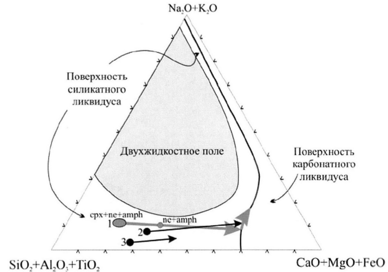
Рис. 11. Гипотетический тренд позднестадийной эволюции расплавов в ийолит-уртитовых комплексах Витимской провинции (1) на Хамильтоновской проекции. Траектории дифференциации меллититовых магм (2) и базальтов (3) по (Lee, Wyllie, 1998). Срх – клинохлорит, не – нефелин, амфр – амфибол.
