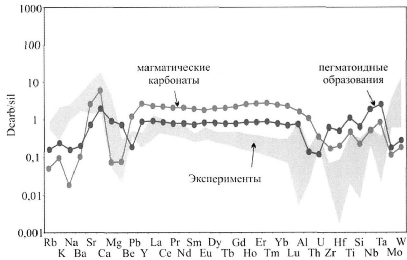
Рис. 12. Карбонатно-силикатные (Dcarb/sil) коэффициенты распределения некоторых редких и редкоземельных элементов между кальцитами, пегматоидными амфибол-нфелин-кальцитовыми обособлениями и щелочными магматическими силикатными породами Витимской провинции и их сопоставление с экспериментальными данными: Hamilton et al., 1989; Kjarsgaard, 1998; Veksler et al., 1998, 2012; Veksler, Lentz, 2006.
