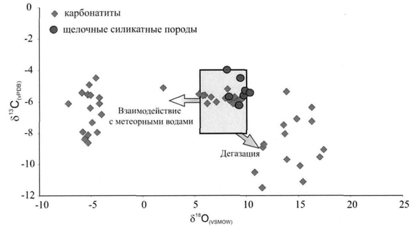
Рис. 15. Изотопные составы С и О в карбонатах из пород карбонатитовых комплексов Юго-Западного Забайкалья. Область первичных карбонатов (PIC) и тренды изменения изотопных составов по (Demeny et al., 2004).
