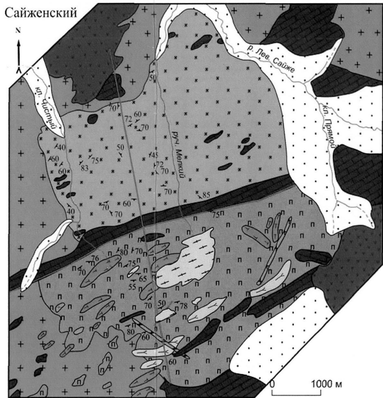
Рис. 4. Схемы геологического строения некоторых массивов Витимской провинции (по данным А.О. Шаракшинова, 1984). 1 – современные рыхлые отложения; 2 – известняки; 3 – сланцы; 4 – габброиды; 5 – пироксениты; 6 – ийолиты; 7 – уртиты; 8 – нефелиновые сиениты; 9 – щелочные сиениты; 10 – граниты; 11 – дайки аплитовидных гранитов; 12 – порфириновые граниты; 13 – линии тектонических нарушений: а – достоверные, б – предполагаемые; 14 – элементы залегания.
