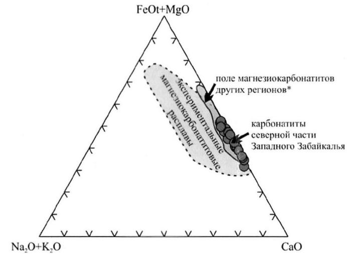
Рис. 9. Диаграмма системы FeO+MgO-(Na,K)_2O-CaO для карбонатитов северной части Западного Забайкалья и мантийных магнезиокарбонатитов других регионов* (Векуско Лейк (Chakhmouradian et al., 2009) и Снап Лейк в Канаде (Agashev et al., 2008), Невания в Индии (Viladkar, 1998; Doroshkevich et al., 2010 b), Дорова, Шава (Harmer et al., 1998), Часвета (Bailey, 1989), Тамазерт (Mourtada et al., 1997) и Шпитцкоп в Африке (Harmer, 1999), Пенченга в России (Врублевский и др., 2003 б). Область экспериментальных первичных карбонатных расплавов, равновесных с перидотитом по (Ionov et al., 1998; Klemme et al., 1995; Sweeney et al., 1995; Foley et al., 2009; Dasgupta et al., 2009).
