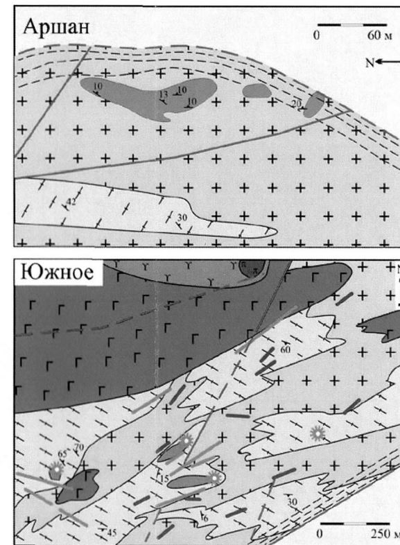
Рис. 7. Схемы геологического строения Халютинского месторождения, Аршанского и Южного проявлений карбонатитов по (Мауришин и др., 1976; Карбаинов и др., 1979; Рипп и др., 2000). 1 –алевриты, песчаники, аргиллиты (K); 2 –биогитовые, амфибол-биогитовые разнотельные граниты, граносиениты, кварцевые диориты, гнейсограниты (PZ 1 ); 3 – перидотиты (PZ 2 ); 4 – анортозиты; 5 – амфибол-пироксеновое габбро (PZ 3 ); 6 – 8 – карбонатиты: 6 – участки площадного распространения карбонатитов, 7 – трубообразные тела, 8 – жильные тела; 9 – граниты, кварцевые сиениты; 10 – дайки шпонкинитов и щелочных сиенитов; 11 – зоны расщелачивания; 12 – линии тектонических нарушений: а – достоверные, б – предполагаемые; 13 – элементы залегания; 14 – участки проявления карбонатитов на Халютинском месторождении: (1) Халютинский, (2) Верхне-Халютинский, (3) Нижне-Шалутайский, (4) Верхне-Шалутайский, (5) Аршан-Халютинский; 15 – линия разреза; 16 – скважины.
