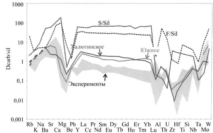
Рис. 14. Сопоставление коэффициентов распределения элементов между карбонатной и силикатной фазами (Dcarb/sil) для пород Халютинского месторождения и Южного проявления с результатами экспериментальных исследований (Hamilton et al., 1989; Kjarsgaard, 1998; Veksler et al., 1998, 2012; Сук, 2003; Schultz et al., 2004; Veksler, Lentz, 2006). Пунктиром показаны участки графиков, пересчитанных Dcarb/sil для щелочей по составу включений. S/Sil и F/Sil - коэффициенты распределения между несмесимыми сульфатно-силикатной и фторидно-силикатной жидкостями, соответственно (Veksler et al., 2012).
