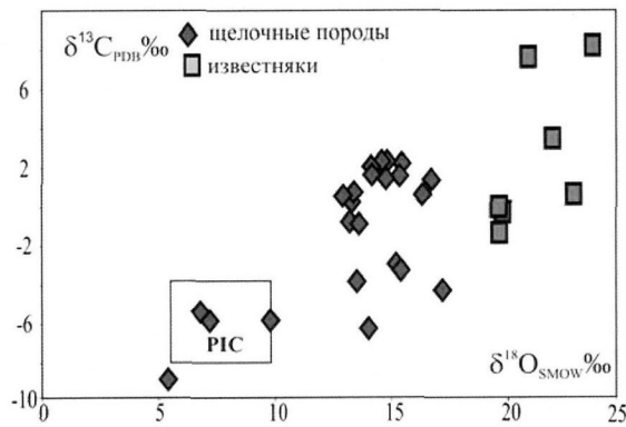
Рис. 13. Соотношение \delta^{13}\text{C} и \delta^{18}\text{O} для минералов из щелочных магматических силикатных пород и известняков Витимской провинции. Область первичных карбонатов (PIC) по (Demeny et al., 2004).
