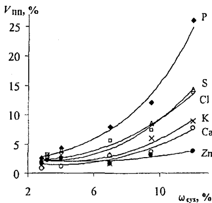
Рис. 3. Зависимость погрешности V_{пп} от массовой доли сухого вещества в молоке
