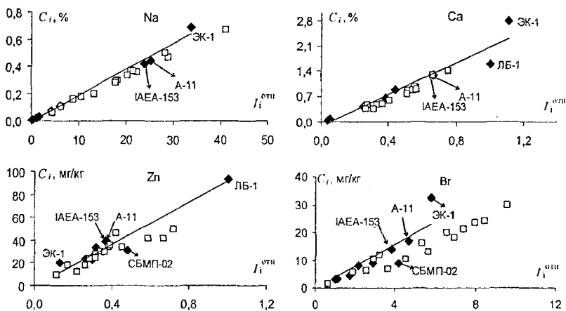
Рис. 2. Зависимость концентрации C_i от интенсивности I_i^Э (—■— градуировочные образцы; —□— молочные продукты)
