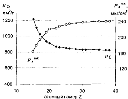
Рис. 4. Зависимость величин \mu_{\Sigma} (■) и P_s^{mk} (○) от Z аналита
