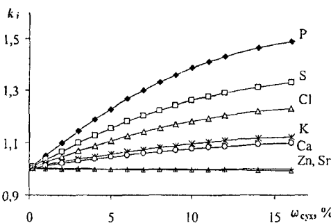
Рис. 5. Зависимость коэффициента k_i от массовой доли сухого вещества в пробе
