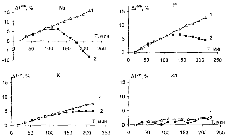
Рис. 1. Относительное изменение интенсивностей K\alpha -линий Na, P, K и Zn за время облучения T (1 – обезжиренное молоко, 2 – жирное молоко)
