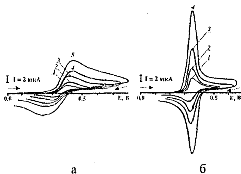
Рис. 3. Циклические вольтамперные кривые 1 \cdot 10^{-3} моль-дм ^{-3} гидрохинона в 0.1 М НСl на графито-эпоксидном электроде в пассивном (а) и активированном (б) состояниях; v , В·с ^{-1} : 0.002 (1); 0.005 (2); 0.01 (3); 0.02 (4), 0.05 (5).
