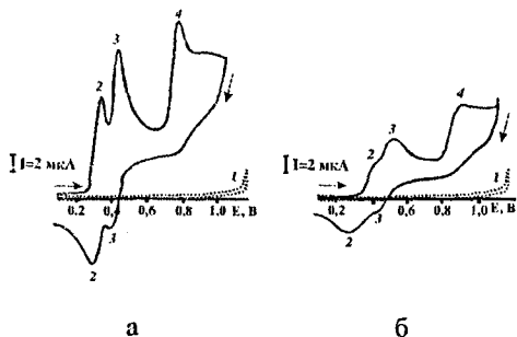
Рис. 6. Циклические вольтамперные кривые диоксибензолов в 0.1 М НСl на графито-эпоксидном электроде в активированном (а) и пассивном (б) состояниях: 1 – фоновая кривая; 2 – гидрохинон; 3 – пирокатехин; 4 – резорцин ( c_0 = 1 \cdot 10^{-3} моль·дм -3 , v = 0.01 \text{ В} \cdot \text{с}^{-1} ).
