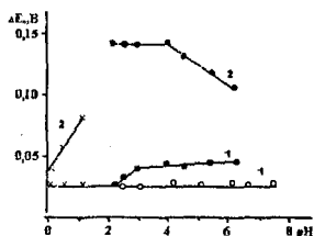
Рис. 5. Зависимость \Delta E_p систем гидрохинон/ n -бензохинон и пирокатехин/ o -бензохинон от pH в 0.1–1.0 М HCl («1X» и «2X»), универсальных буферных растворах Бриттона-Робинсона (0.04 М: H_3BO_3 + H_3PO_4 + CH_3COOH ; «1•» и «2•») и МакИлвейна (0.1 М лимонная кислота + 0.2 М Na_2HPO_4 ; «1O») на графито-эпоксидном электроде в активированном (1) и пассивном (2) состояниях ( c = 1 \cdot 10^{-3} моль·дм -3 , v = 0.01 В·с -1 ).
