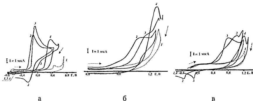
Рис. 1. Циклические вольтамперные кривые диоксибензолов на механически обновляемом никелевом электроде в 0.05 М KOH (а); 0.05 М H 2 SO 4 (б); 0.10 М Na 2 SO 4 (в): 1 – фоновая кривая; 2 – гидрохинон; 3 – пирокатехин; 4 – резорцин ( c_0 = 7 \cdot 10^{-3} моль-дм -3 , \nu = 0.1 В·с -1 ).
