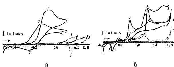
Рис. 1. Циклические вольтамперные кривые диоксибензолов на механически обновляемом никелевом электроде в 0.05 М KOH (а); 0.05 М H 2 SO 4 (б); 0.10 М Na 2 SO 4 (в): 1 – фоновая кривая; 2 – гидрохинон; 3 – пирокатехин; 4 – резорцин ( c_0 = 7 \cdot 10^{-3} моль-дм -3 , \nu = 0.1 В·с -1 ).
