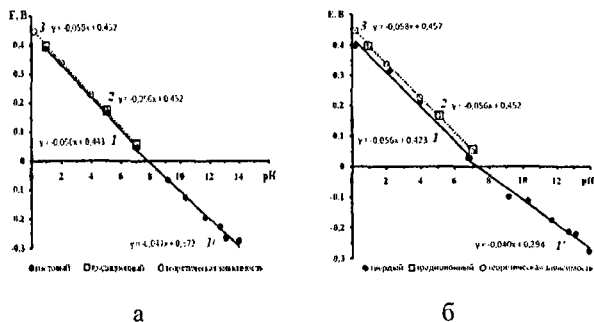
Рис. 8. Зависимость величины потенциала E_i от значения pH раствора для пастового (а, прямые 1, 1'), твёрдого (б, прямые 1, 1'), «традиционного» (2) хингидронных электродов и теоретически рассчитанные значения (3).
