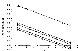
Рис. 7. Зависимость потенциалов анодных (1 – 3) и катодных (1', 2'), пиков гидрохинона (1, 1'), пирокатехина (2, 2') и резорцина (3) от pH буферных растворов ( c_0 = 1 \cdot 10^{-3} моль·дм -3 , \nu = 0.01 В·с -1 ).
