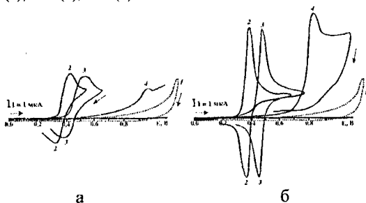
Рис. 4. Циклические вольтамперные кривые диоксибензолов на пассивном (а) и активированном (б) графито-эпоксидном электроде в 0.1 М НСl: 1 – фоновая кривая; 2 – гидрохинон; 3 – пирокатехин; 4 – резорцин ( c_0 = 1 \cdot 10^{-3} моль-дм ^{-3} , v = 0.01 В·с ^{-1} ).
