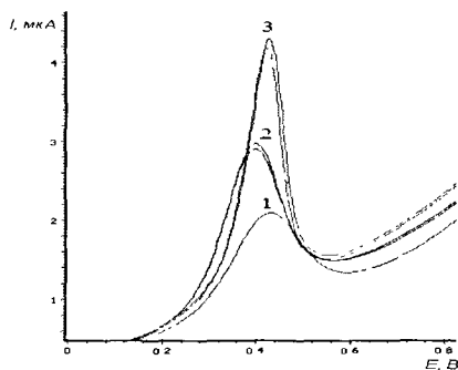
Рис. 8. Вольтамперограммы электроокисления осадков палладия, полученных из растворов, содержащих: 1. - C_{Pd^{2+}} = 0,1 мг/л; 2. - C_{Pd^{2+}} = 0,1 мг/л + щавелевая кислота; 3. - после 10 мин. УФО раствора, содержащего C_{Pd^{2+}} = 0,1 мг/л + щавелевая кислота.
