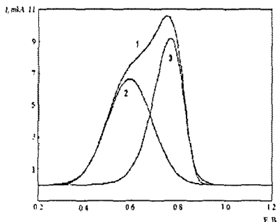
Рис.2 Вольтамперная кривая электроокисления бинарного сплава палладий - золото. Условия экспериментов: C_{Au^{3+}} = 0,05 \text{ мг/дм}^3 ; C_{Pd^{2+}} = 0,03 \text{ мг/дм}^3 . 1 - вольтамперная кривая до разделения пиков; 2 - анодный пик палладия, выделенный из суммарной кривой; 3 - анодный пик золота, выделенный из суммарной кривой.
