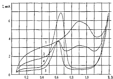
Рис. 7. Вольтамперные кривые электроокисления осадков Au - Pd, полученных из растворов, содержащих: 1. - C_{Au^{3+}} = 0,2 мг/л; 2. - C_{Au^{3+}} = 0,2 мг/л + C_{Pd^{2+}} = 0,1 мг/л; 3. - после 20 мин. УФО раствора, содержащего C_{Au^{3+}} = 0,2 мг/л + C_{Pd^{2+}} = 0,1 мг/л; 4. - после добавки C_{Pd^{2+}} = 0,1 мг/л.
