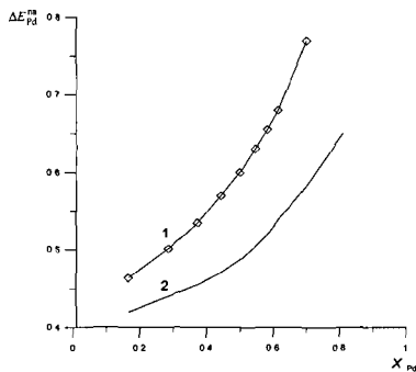
Рис. 5. Величина смещения потенциалов анодных пиков палладия как функция мольной доли палладия в электролитическом сплаве с золотом: 1– кривая построенная по экспериментальным данным, 2– кривая построенная по формуле 2.
