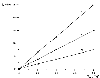
Рис. 6. Зависимость тока анодного пика палладия от концентрации ионов палладия(II) в растворе после фотохимического восстановления золота(III) в присутствии органических кислот: 1 – щавелевая кислота, 2 – муравьиная кислота, 3 – лимонная кислота.
