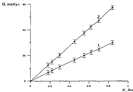
Рис. 3. Зависимость площади под анодным пиком золота (кривая 1) и суммарным анодным пиком (кривая 2) от мольной доли золота в электролитическом осадке Au – Pd. Условия опыта: фон 0,1 М HCl, W = 60 мВ/сек, C_{Au^{+3}} = 0,01 - 0,10 мг/дм 3 , C_{Pd^{+2}} = 0,02 мг/ дм 3 , t_s = 120 с.
