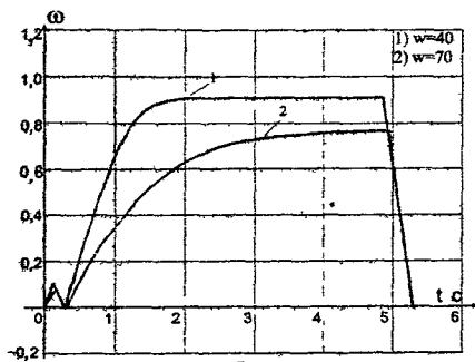
Рис. 4 Процесс работы в течение одного включения с выбором слабину кавата при t_{\text{вкл}}=5,3 с
