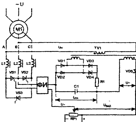
Рис 1 Схема дроссельного регулируемого электропривода
