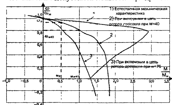
Рис. 5. Механические характеристики электропривода
