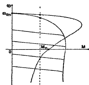
Рис. 10. Механические характеристики электропривода
