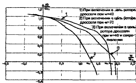
Рис. 7. Механические характеристики
