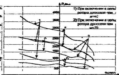
Рис. 8. Изменение потерь в электродвигателе при дроссельном регулировании
