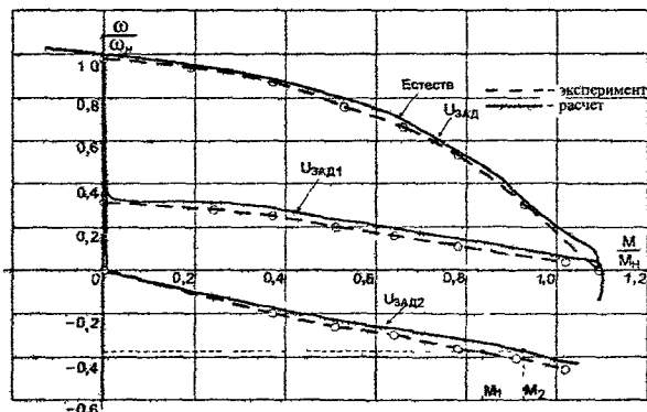
Рис. 3 Расчетные и экспериментальные механические характеристики электропривода
