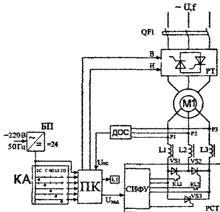
Рис 14 Функциональная схема электропривода
