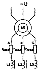
Рис. 9. Схема включения дросселя и добавочного сопротивления
