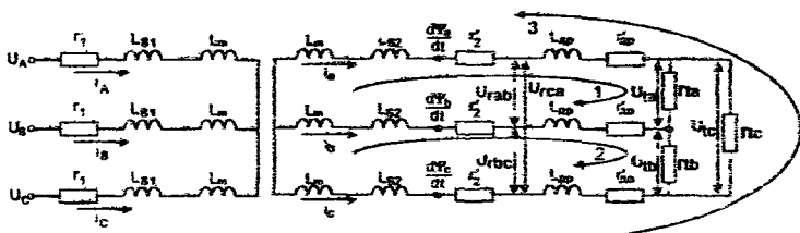
Рис. 2. Схема замещения с учетом допущений
