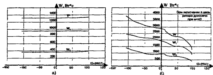
Рис. 6. Изменение потерь энергии в электродвигателе при включении в цепь ротора сопротивления (а) и дросселя (б)
