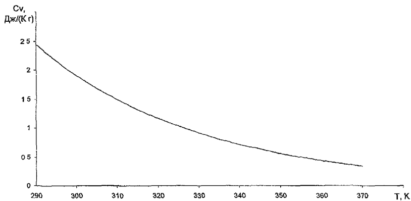
Рис 5 График зависимости теплоемкости полиметилметакрилата от температуры
