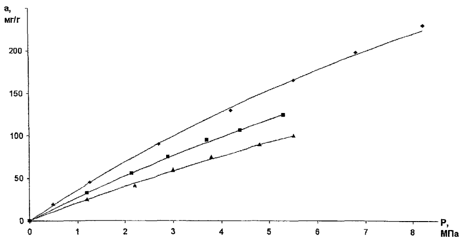
Рис 2 Изотермы сорбции \text{CO}_2 полиметилметакрилатом (PMMA) для температур ◆ – T = 306 \text{ K} , ■ – T = 315 \text{ K} , ▲ – T = 332 \text{ K} Точки - экспериментальные данные, кривые – результаты расчета
