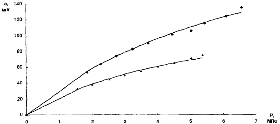
Рис 1 Изотермы сорбции \text{CO}_2 поликарбонатным полимерным сорбентом ◆ – T = 308\text{K} , ▲ – T = 318\text{K} Точки - экспериментальные данные, кривые – результаты расчета по предложенной модели
