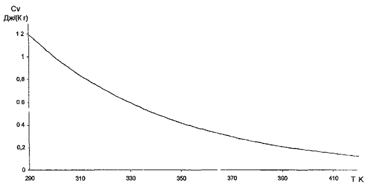
Рис 7 График зависимости теплоемкости поликарбоната от температуры
