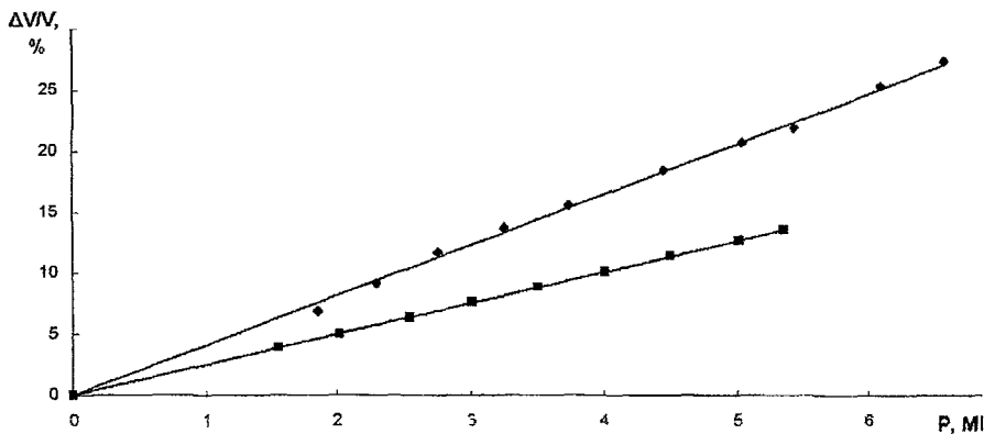
Рис 3. Экспериментальные изотермы относительной объемной деформации поликарбоната (PC) при сорбции \text{CO}_2 ■ – T = 318\text{K} , ◆ – T = 308\text{K}
