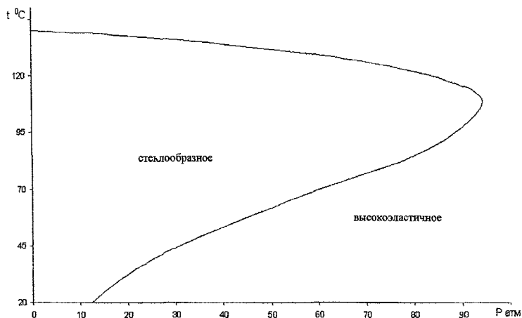
Рис 6 Граница области стеклообразного состояния поликарбоната, взаимодействующего с диоксидом углерода
