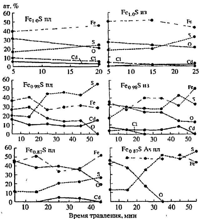
Рис 5 Профили концентраций элементов вглубь кристаллов пирротина различного состава пластинчатой и изометричной формы по данным оже-спектроскопии с ионным травлением
