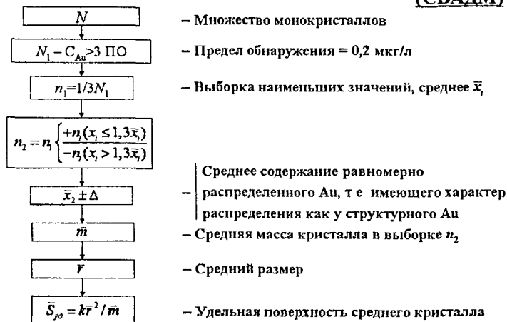
Рис 2 Принципиальная схема разделения форм золота и выделения структурной формы по методу СВАДМ
