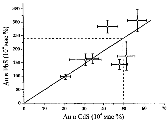
Рис 4 Диаграмма фазового соответствия системы CdS–PbS–Au при 500°C и давлении 1 кбар Коэффициент распределения \bar{K}_{Au}^{Gr/Gr} = 4,7 \pm 1,1
