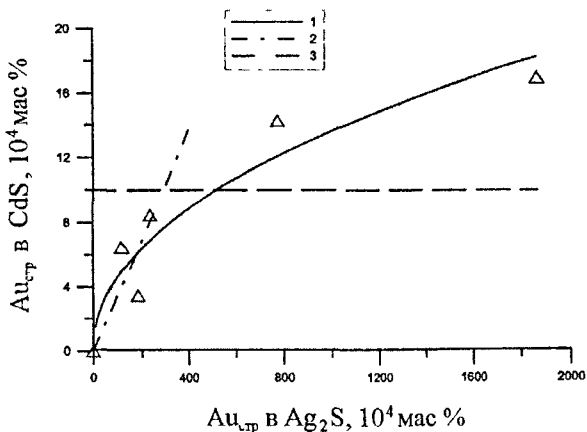
Рис. 6. Распределение структурной примеси Au между CdS и Ag 2 S при 450°C и давлении 1 кбар (по результатам СВАДМ) 1 – аппроксимация экспериментальных данных, 2 – линейная аппроксимация точек < 10^3 мас % Au в CdS ( K_{Au}^{Cr/Ag} \sim 0,03 ), 3 – предел вхождения Au в CdS [6, 7]
