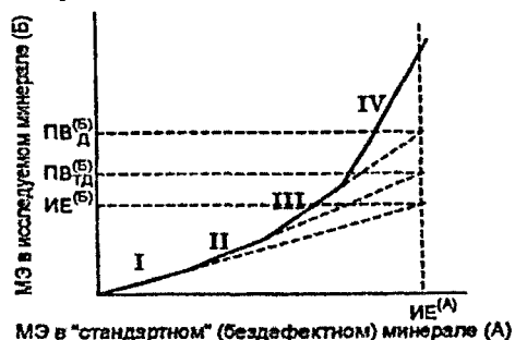
Рис 1 Схематическое представление распределения микроэлемента между «стандартным» (условно бездефектным) кристаллом и исследуемым кристаллом, содержащим несколько типов дефектов кристаллической структуры, при возрастающей концентрации микроэлемента в системе (по [1])
