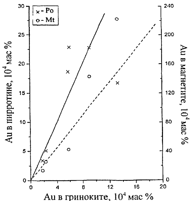
Рис 3 Распределение структурной примеси золота между сосуществующими фазами стехиометрическим пирротинном, магнетитом и гринокитом
