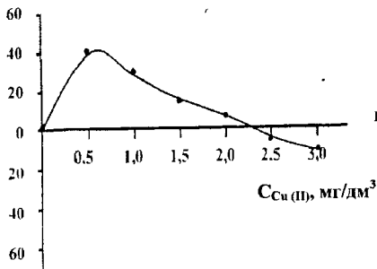
Рис. 6. Зависимость систематической погрешности определения Cu(II) от ее концентрации в растворе в присутствии Se(IV)
