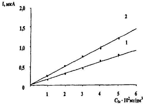
Рис. 2. Зависимость катодного тока \text{Se(IV)} от его концентрации в растворе.
