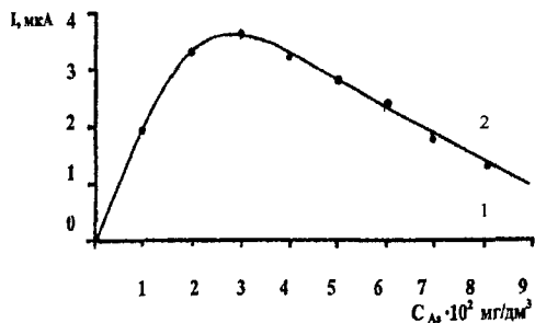
Рис. 4. Зависимость катодного тока As(III) от его концентрации в растворе.
