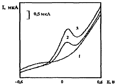
Рис. 7. Вольтамперограммы аналитических сигналов As(III) на ЗГЭ в растворе сахара в присутствии растворенного кислорода без пробоподготовки. фон – 0,1М Трилон Б; E_n = -1,0 В; \tau_n = 60 с; 1– фон; 2– проба; 3– проба с добавкой.
