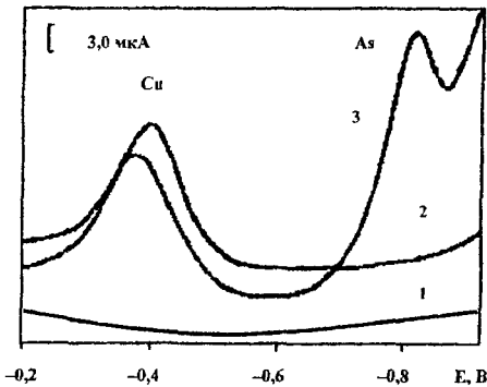
Рис. 3. Вольтамперограммы \text{Cu(II)} и \text{As(III)} в системе \text{As-Cu-Hg}
