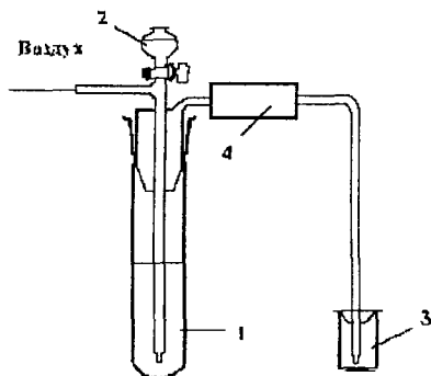
Рис. 8. Установка для отгонки мышьяка в виде AsCl_3
