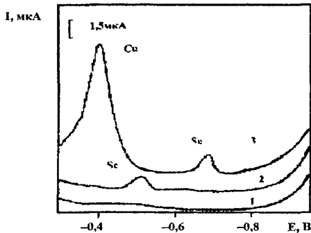
Рис. 1. Вольтамперограммы \text{Se(IV)} и \text{Cu(II)} в системе \text{Se-Cu-Hg} фон - 0,6 \text{ M HCl} + 5 \text{ мг/дм}^3 \text{ Hg(II)} ; E_n = -0,2 \text{ В} ; \tau_n = 60 \text{ с} 1- фон; 2 - фон + 0,02 \text{ мг/дм}^3 \text{ Se(IV)} ; 3 - фон + 0,02 \text{ мг/дм}^3 \text{ Se(IV)} + 2 \text{ мг/дм}^3 \text{ Cu(II)}
