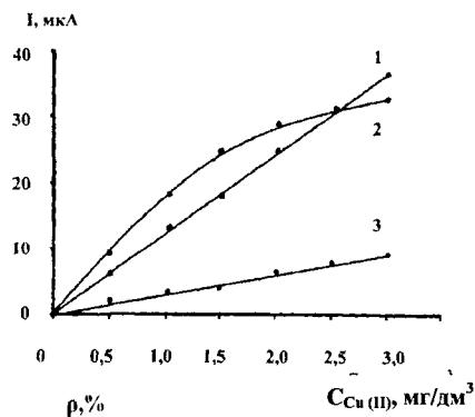
Рис. 5. Зависимость катодного тока электровосстановления Cu(II) от ее концентрации в растворе.
