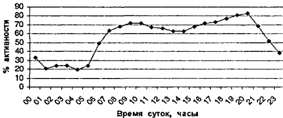
Рис. 1. Распределение суточной активности бурого медведя
