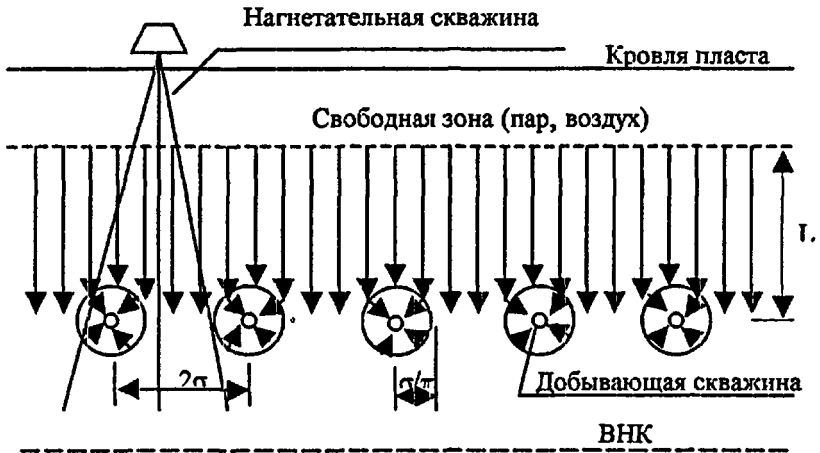
Рис. 7. Принципиальная схема вертикальной фильтрации жидкости при геомошактной разработке L – расстояние от свободной зоны до подземных скважин 2\sigma – расстояние между добывающими скважинами
