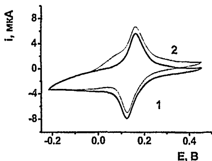
Рисунок 3. Вольтамперограмма, полученная с помощью АХЭ/БЛ сенсора до (1) и через 3 мин. после введения 1.5 мМ АТТХ (2)
