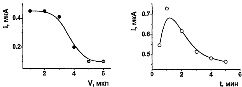
Рисунок 1. Влияние объема 0.5% суспензии нафиона, наносимой на электрод, (1) и продолжительности кросс-сшивки БуХЭ парами глутарового альдегида (2) на сигнал биосенсора на 0.1мМ БуТХИ
