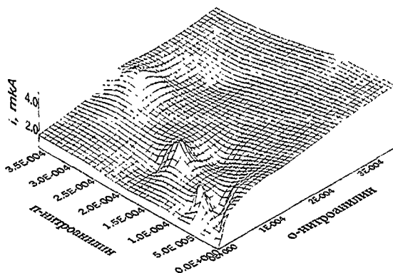
Рисунок 8. Моделирование сигнала пероксидазного сенсора в смеси n - и o -нитроанилина по 50 экспериментальным значениям отклика. Программа Surfer.
