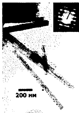
Рис.4. Электронная микрофотография (ПЭМ) образца 6-НС-3.
