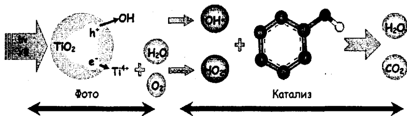
рис. 3. схема процесса фотокаталитической реакции на диоксиде титана.
