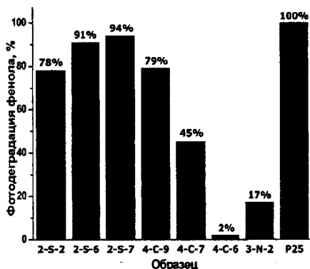
Рис. 6. Степень фотодеградации фенола после 90 мин УФ облучения
