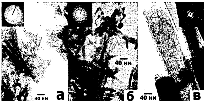
Рис. 2. Электронные микрофотографии (ПЭМ) и ЭД (вставка) образцов 5-НТ-1 - (а), 5-НТ-4 - (б) и 5-НТ-6 - (в).
