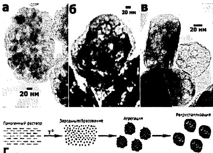
Рис. 1. Электронные микрофотографии (ПЭМ) образцов 4-C-7 - (а), 4-C-8 - (б), 4-C-9 - (в) и схема образования наночастиц мезопористого анатаза.
