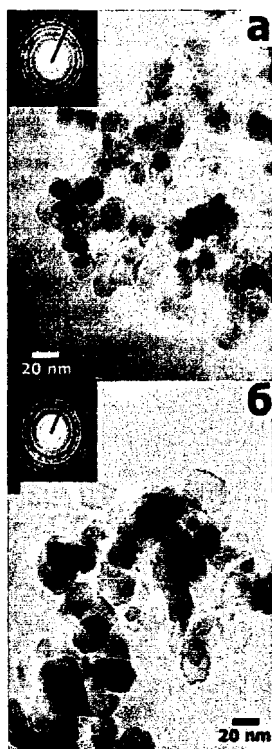
Рис. 9. Электронные микрофотографии (ПЭМ) образцов 7-ЗГ-1 (а) и 7-ЗГ-4 (б).
