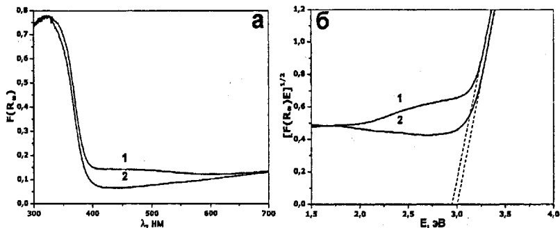
Рис. 10. Спектры диффузного отражения (а) и зависимость функции преобразования Кубелка-Munk от энергии абсорбированного света (б) образцов 7-ЗГ-1 (1) и 7-ЗГ-2 (2).
