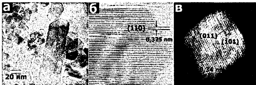
Рис. 8. (а) Электронная микрофотография (ПЭМВР) образца 2-S-7 ; (б) Электронная микрофотография (ПЭМВР) слоев частицы рутила, взятой с рис. 8а; (в) Электронная микрофотография (ПЭМВР) слоев частицы анатаза, взятой с рис. 8а.
